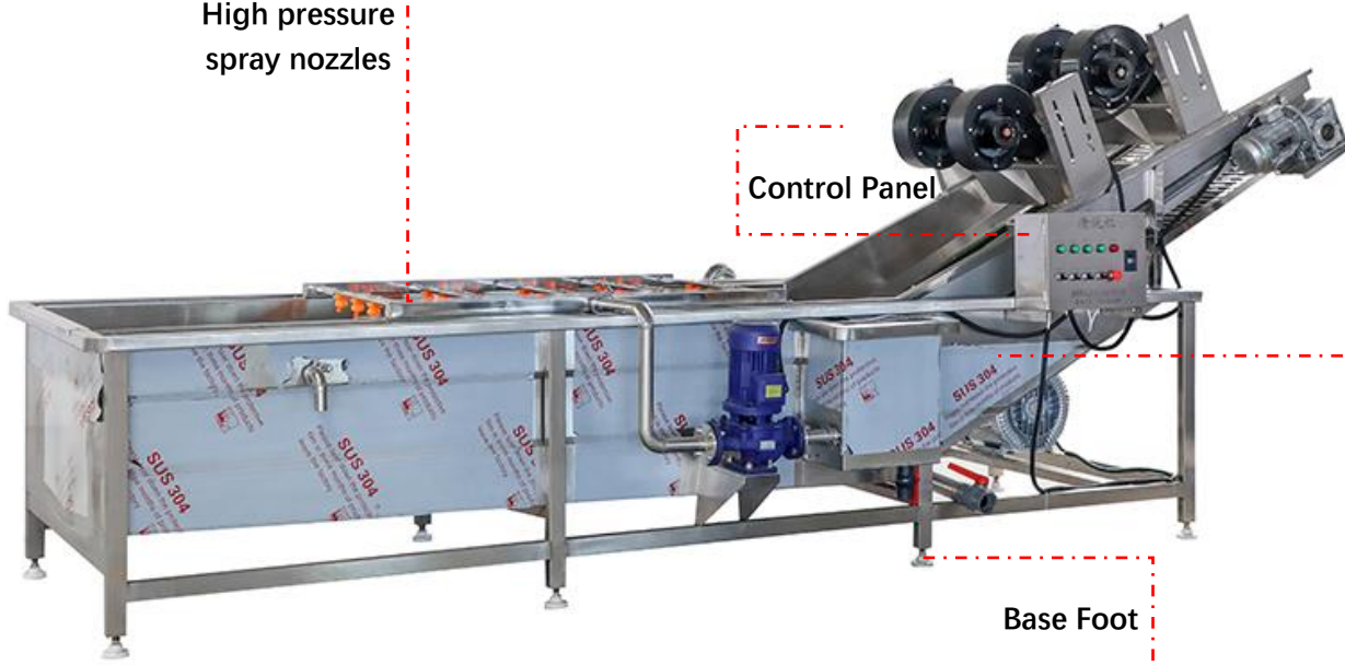
SUS 304 stainless steel machine body
